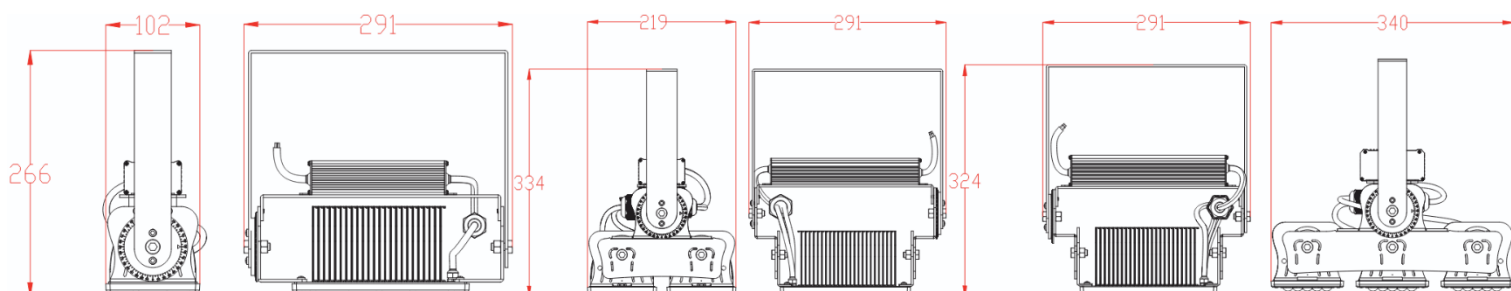
FAFFL-100W
